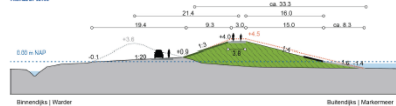
MAATGEVEND PROFIEL WARDER 2 (SECTIE HE-9 VANAF DUKPAAL 52 TOT 62+50) PROFIEL DP 53+40
