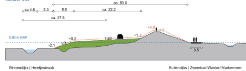
MAATGEVEND PROFIEL WARDER 1 (SECTIE HE-9 VAN DUKPAAL 48+50 TOT 52) PROFIEL DP 53+40
