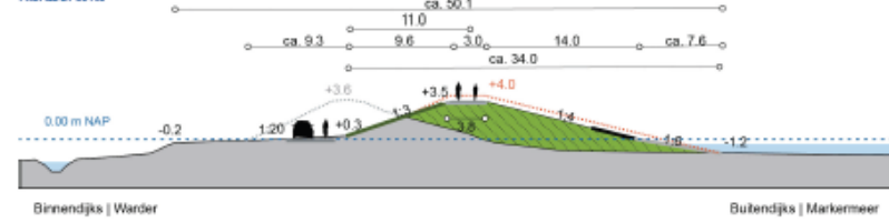
MAATGEVEND PROFIEL WARDER 2 (SECTIE HE-9 VANAF DUKPAAL 52 TOT 62+50) PROFIEL DP 53+40
