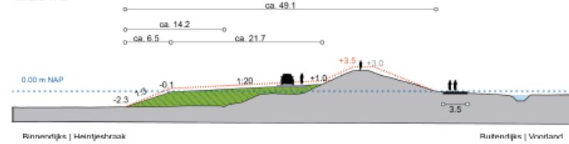
MAATGEVEND PROFIEL HEINTJESBRAAK 2 (SECTIE HE-8 VAN DUKPAAL 44+50 TOT 46+50) PROFIEL DP 45+40
